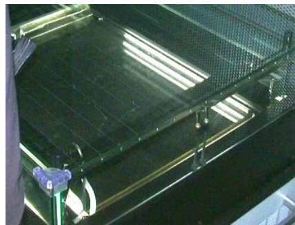
Částice za sebou zanechávají kondenzační čáry jako letadla.
