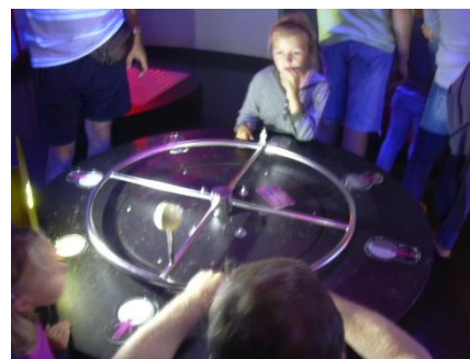
Kterak vznikají měsíční fáze
